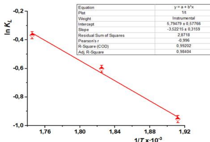
2-rasm. \ln K_L ning 1/T ga bog‘liqligi grafigi
