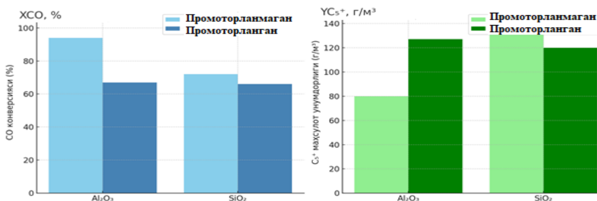
2-расм. T = 200 °C да CO ва H_2 дан углеводородлар синтезида CO конверсияси ( X_{CO} , %) ва C_5^+ маҳсулотлар унуми ( Y_{C_5^+} , г/м 3 ) га 20%Co–20%Fe–5%B–1.5%Zr(0–2)%Na/ Al_2O_3 ва 20%Co–20%Fe–5%B–1.5%Zr(0–2)%Na/ SiO_2 катализаторларининг таъсири
