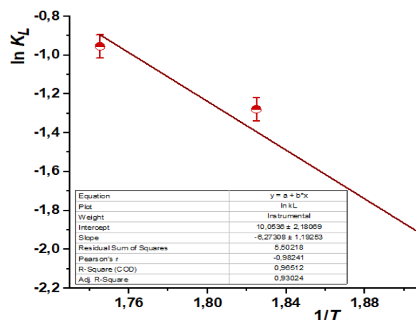
6-rasm. Koks komponentlari uchun \ln K_L ning 1/T ga bog'liqligi grafigi
