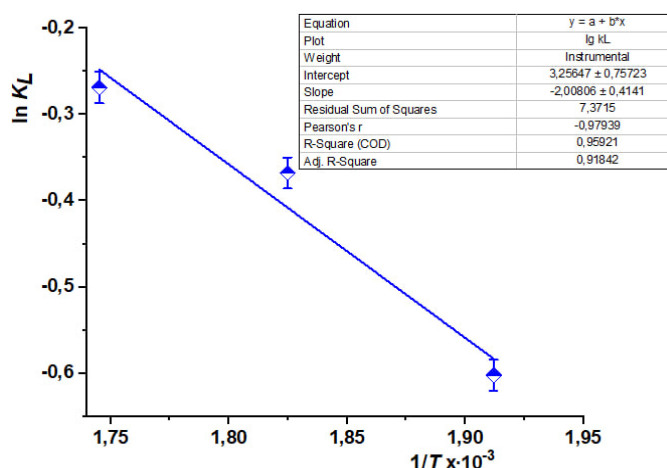
1-rasm. Piroliz jarayonida kinetik konstantaning (KL) haroratga bog‘liqligin
