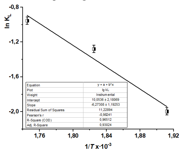
4-rasm. 2–3 halqali aromatik uglevodorodlar uchun \ln K_L ning 1/T ga bog‘liqligi grafigi
