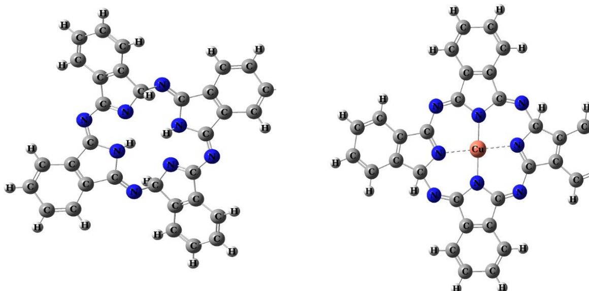
2-rasm. Izoindol ligand va mis saqlagan ftalosianin kompleksining struktura formulalari.
