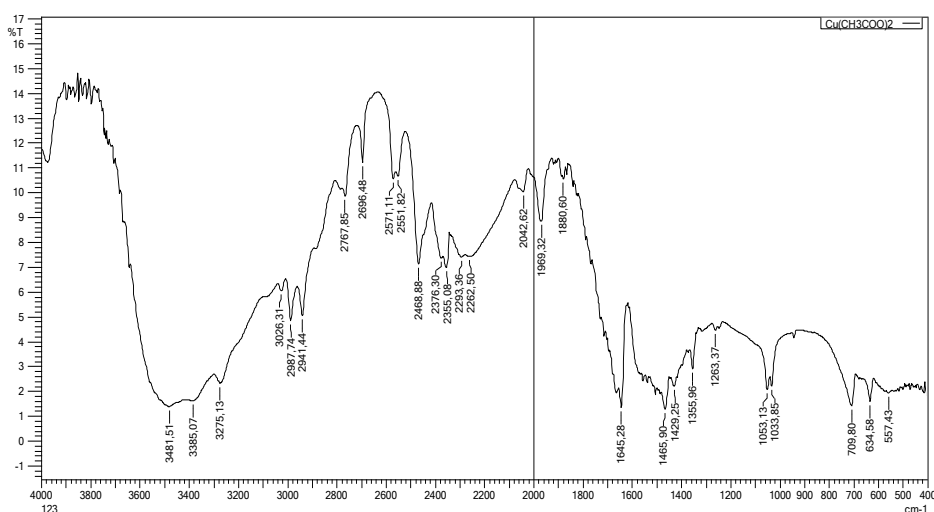
3-rasm. Mis(II) atsetatning IQ-spektroskopiya tasviri
