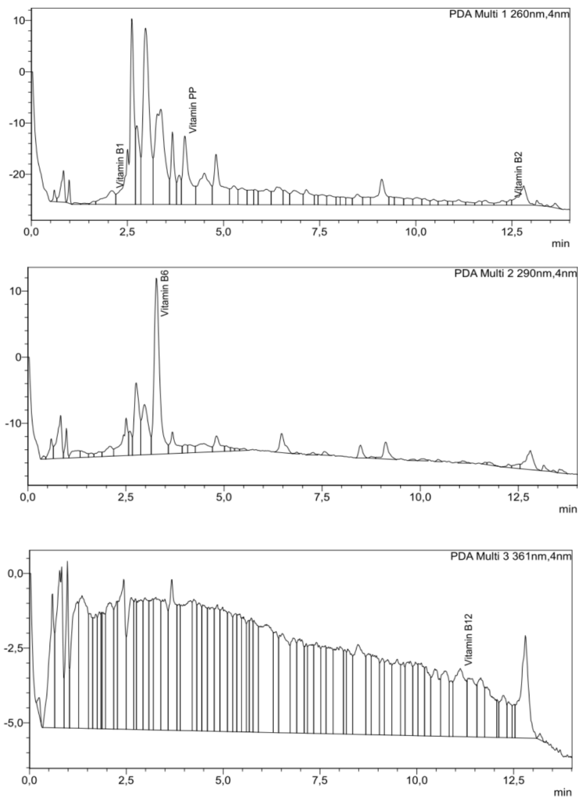
3-rasm. “As-Immun” ekstrakti tarkibidagi B 1 , B 2 , B 6 , B 12 va PP vitaminlar xromotogrammasi
