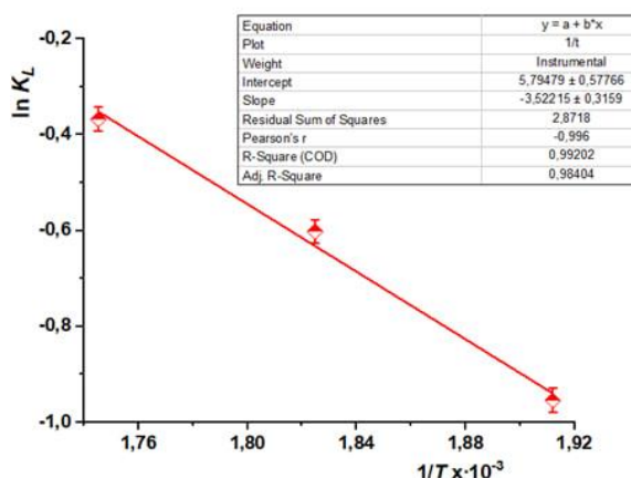
5-rasm. Og'ir neft komponentlari uchun \ln K_L ning 1/T ga bog'liqligi grafigi
