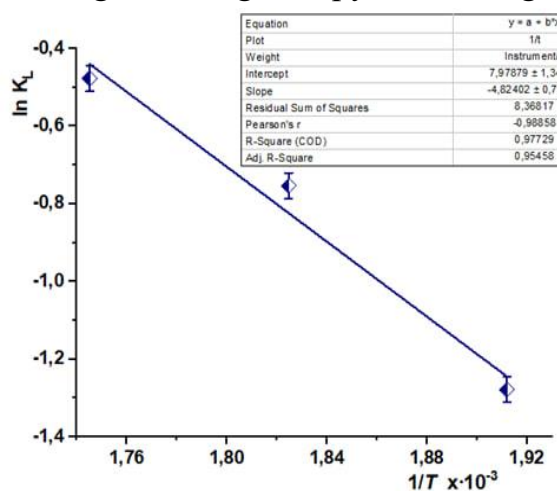
3-rasm. 2–3 halqali aromatik uglevodorodlar uchun \ln K_L ning 1/T ga bog‘liqligi grafigi
