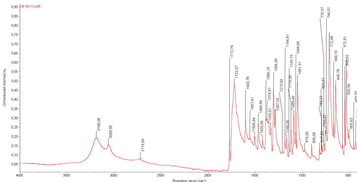
2-rasm. Karboksil guruhi saqlovchi mis ftalosiyanin pigmentining IQ-spektroskopik tahlili
