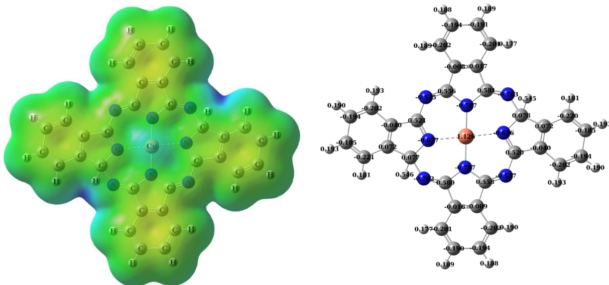
5-rasm. Mis ftalosianin kompleksining ESP (Elektrostatik potensial) molekuladagi elektron zichlik taqsimoti va Mulliken zaryad taqsimoti.
