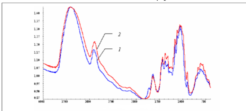
1-rasm. PAS va Na-KMS ning IQ spektri. 1-PAS; 2- NaKMS.
