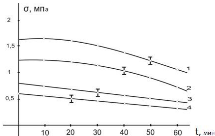
Рисунок 3. Зависимость прочности композиционных материалов от времени хранения при температуре. 1 - 100% гипса; 2 - 90% гипса + 10% керамзита; 3 - 70% гипса + 30% керамзита; 4 - 50% гипса + 50% керамзита.
