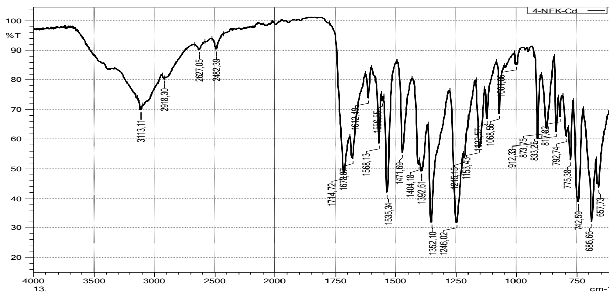
2-rasm. [C_8H_3NO_6]^{2-}Cd^{2+} kompleksining IQ-spektri
