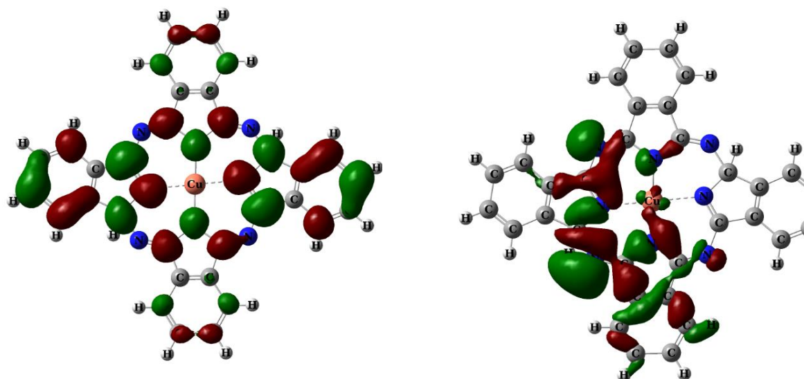
3-rasm. Mis ftalosianin kompleksining HOMO-LUMO energiya darajalari.
