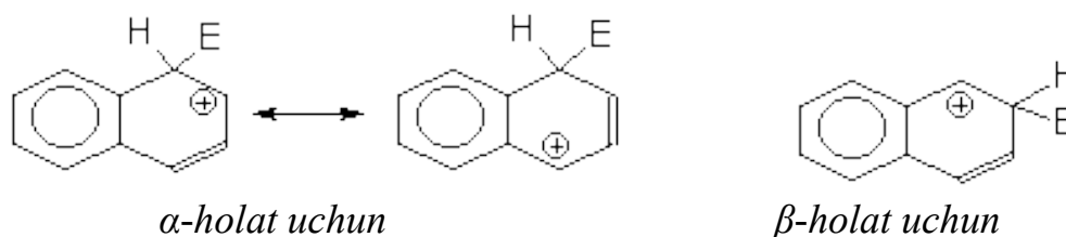
1-rasm. Naftalinning 2 xil holat uchun rezonans tuzilishlari.
