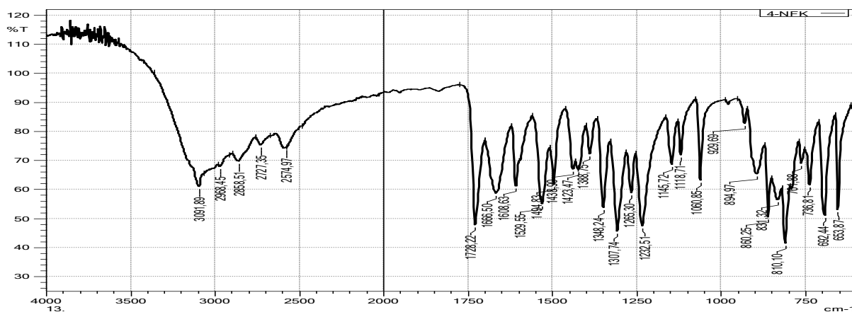
1-rasm 4-nitroftal kislotasining IQ-spektri
