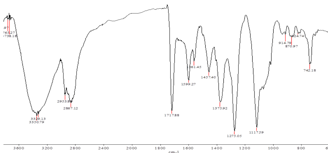
Рис. ИК-спектр продукта конденсации тиокарбамида с формальдегидом.
