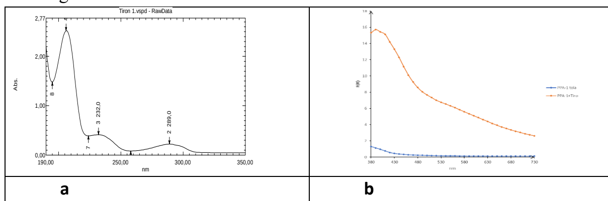
2-Rasm. a) Tironning eritmadagi UV–Vis spektri, b) PPA-1 tolaga immobillangan Tironning nur qaytarish (fluoresensiya) spektri.
