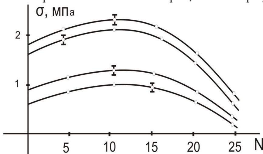
Рисунок 4. Влияние температурного циклирования на прочность композиционных материалов. 1 - 100% гипса; 2 - 90% гипса + 10% керамзита; 3 - 70% гипса + 30% керамзита; 4 - 50% гипса + 50% керамзита.
