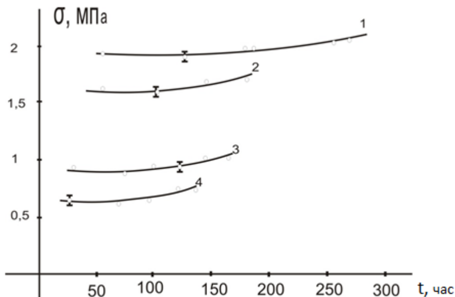
Рисунок 5. Зависимость времени до разрушения прочности композиционных материалов от скорости деформации. 1 - 100% гипса; 2 - 90% гипса + 10% керамзита; 3 - 70% гипса + 30% керамзита; 4 - 50% гипса + 50% керамзита.
