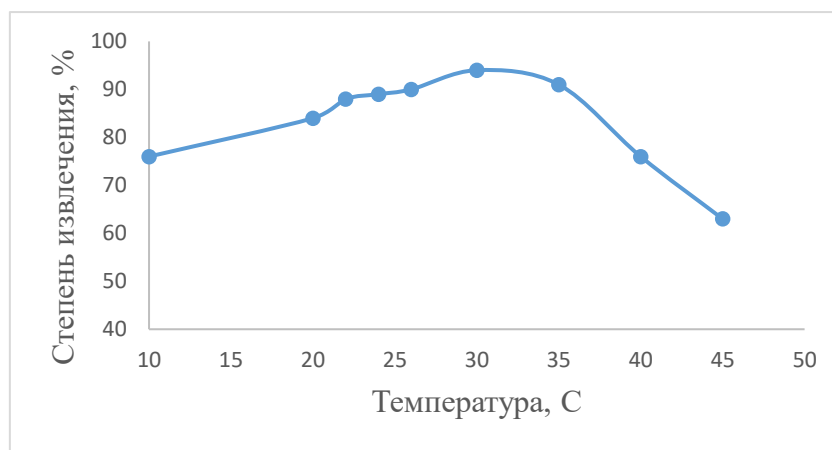
Рис. 1. Влияние температуры на степень извлечения KCl из P3.
