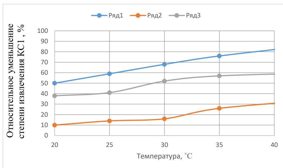
Рис. 3. Влияние температуры раствора и состава н.о. в количестве 5 % от массы солей на относительное уменьшение степени извлечения КС1: 1) глинистые примеси; 2) неглинистые примеси; 3) глинистые примеси : неглинистые примеси в 1:1.
