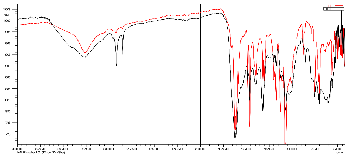
3- rasm. 1-va 2-rasmdagi spektrlar farqi.
