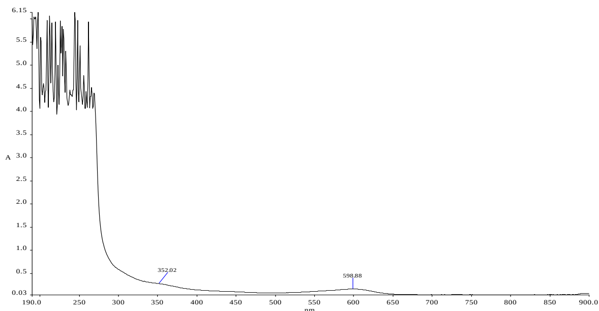
5-rasm. “Indigofera tinctoria L” dan olingan moddaning UF-spektri
