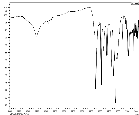
2-rasm. “Isatis tinctoria” dan ajratib olingan indigoning IQ-spektri.
