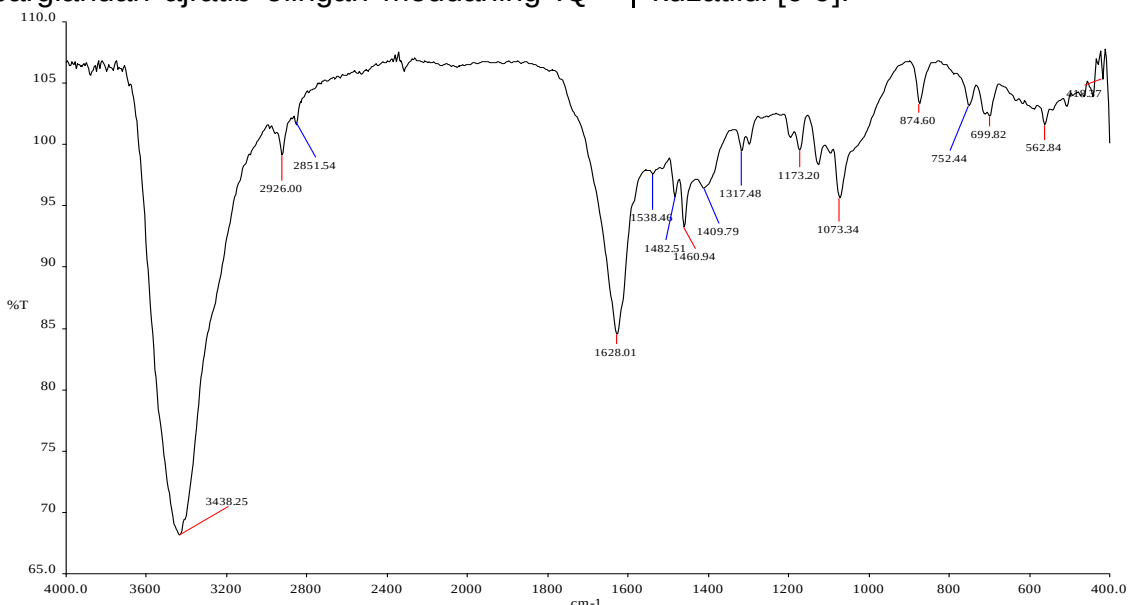
4-rasm. Tajribada “Indigofera tinctoria L” dan ajratib olingan indigoning IQ-spektri.
