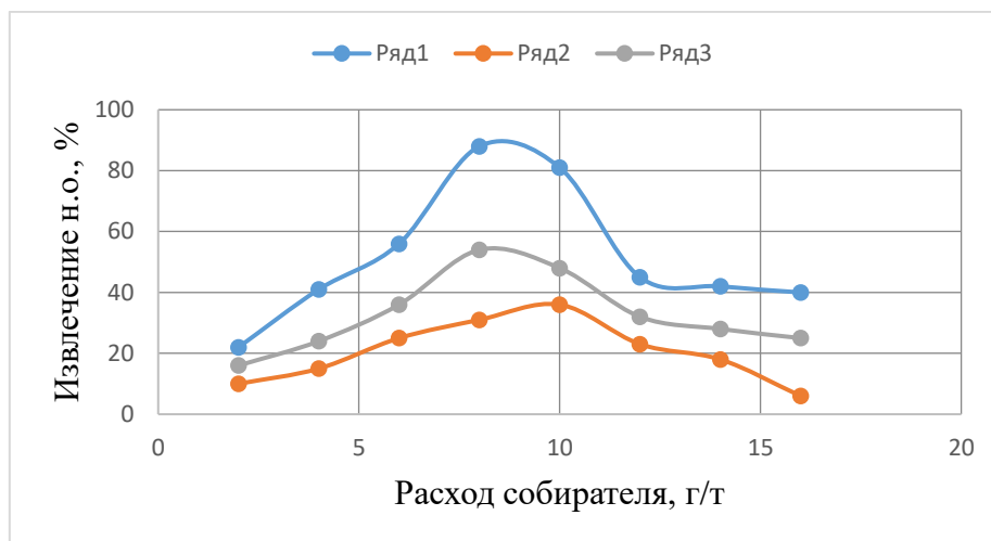
Рис. 4. Влияние расхода собирателя на извлечение н.о. в концентрат (содержание н.о. 5% от массы смеси, температура раствора 22 \pm 1 °C: 1) глинистые примеси; 2) неглинистые примеси; 3) глинистые примеси : неглинистые примеси в 1:1.
