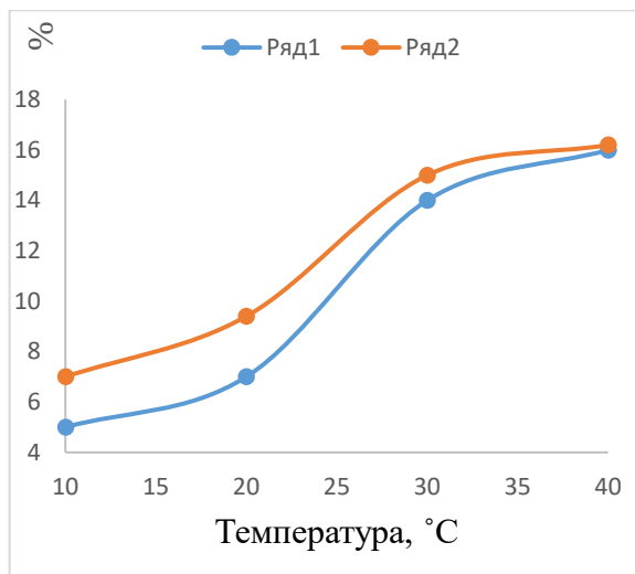
Рис. 7. Влияние температуры раствора и состава н.о. в количестве 5 % от массы солей на относительное уменьшение степени извлечения КС1: а) неглинистые примеси; б) глинистые примеси; 1) ИП; 2) ЖП.
