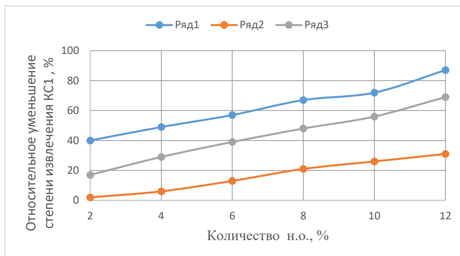
Рис. 2. Влияние количеств н.о. в составе модельного раствора Р3 на относительное уменьшение степени извлечения КС1 ( 20 \pm 1^\circ\text{C} ): 1) глинистые примеси; 2) неглинистые примеси; 3) глинистые примеси:неглинистые примеси в 1:1.
